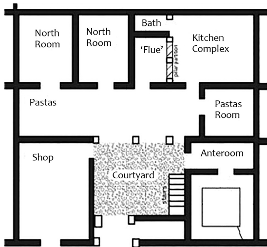
Рис. 6. Тип дома “pastas house” (пастадный дом), план дома в Олинфе V–IV вв. до н.э.
