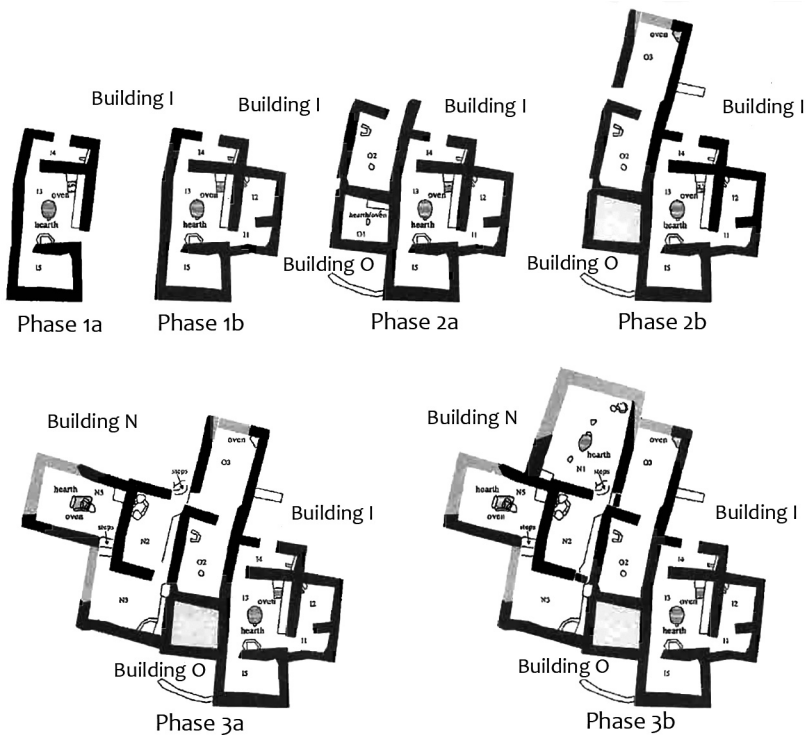
Рис 4. Здание I–O–N во Вронде (XII–XI вв. до н.э.)
