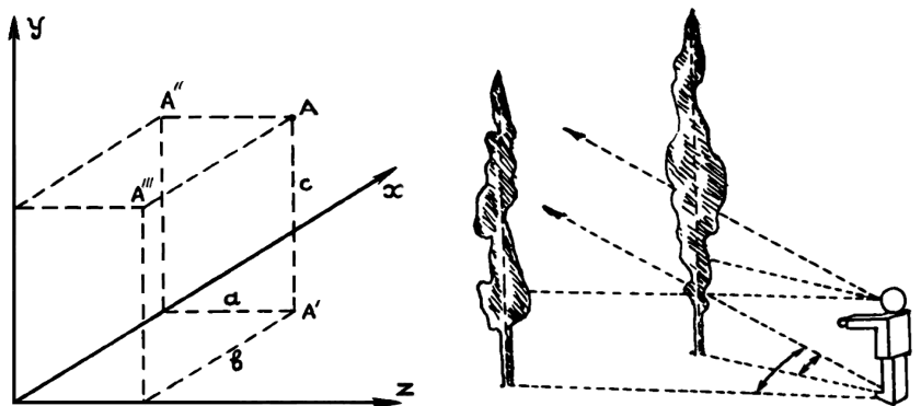
Рис. 1. Декартова и полярная система координат
